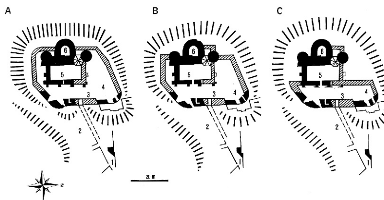
Hypothèses sur l'extension de la « chemise » partielle du donjon.
