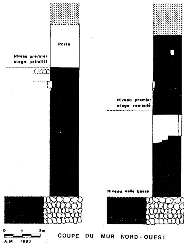
Abaissement du plancher de la salle basse du donjon
